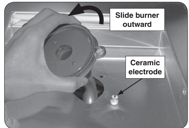
Fig. 33-2 Remove burner
